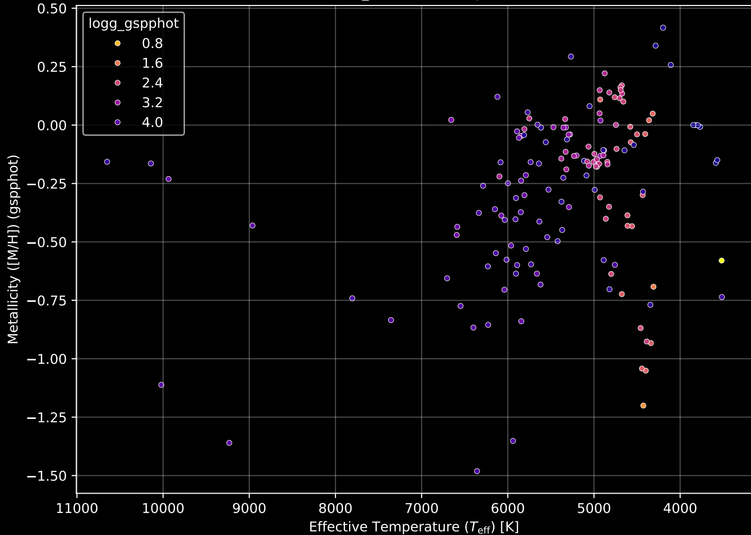
APOGEE DR17 Field: [277-18-O_TESS] Stellar Population Parameters (n= 152)
